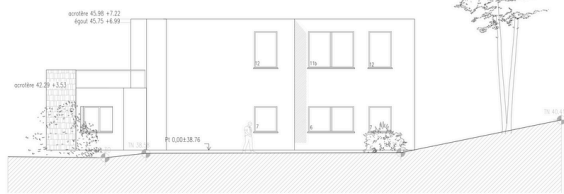
FACADE NORD-EST - PROJET
