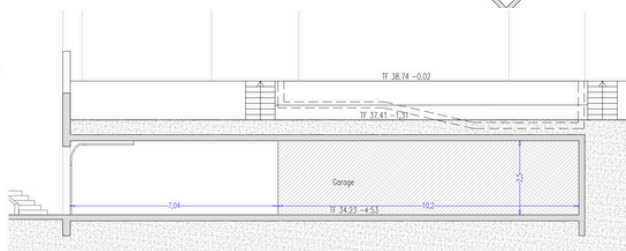
COUPE C
