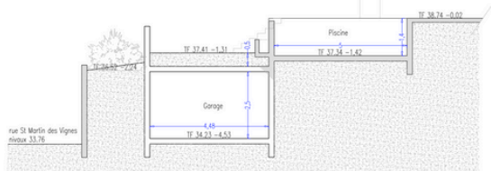
COUPE B
