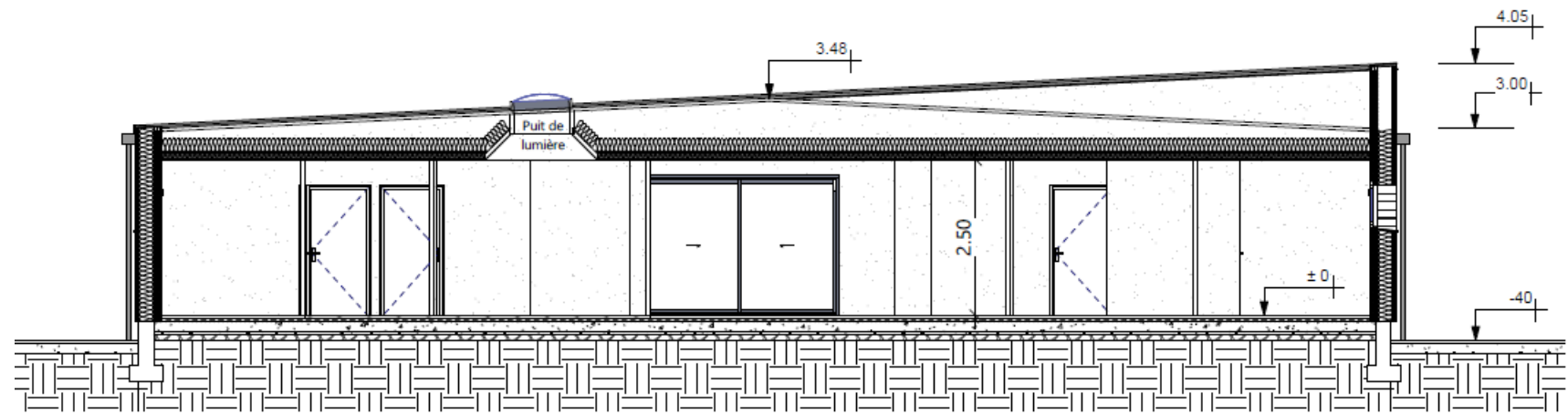
② Coupe Maison Ech : 1 : 75
